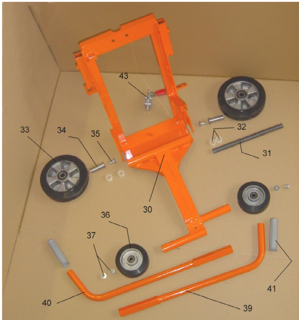
Chassis mit Räder
