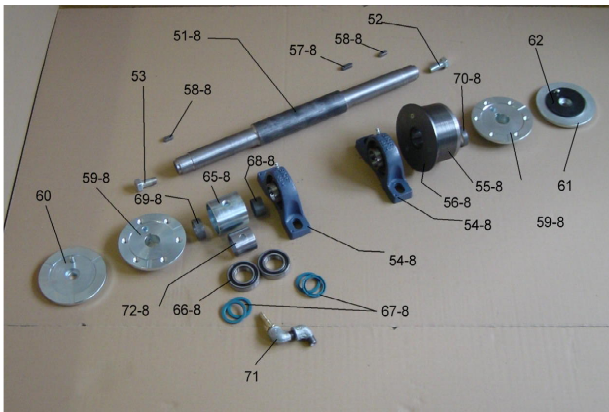
Schneidwelle mit Spülbuchse zu BS6E2-800
