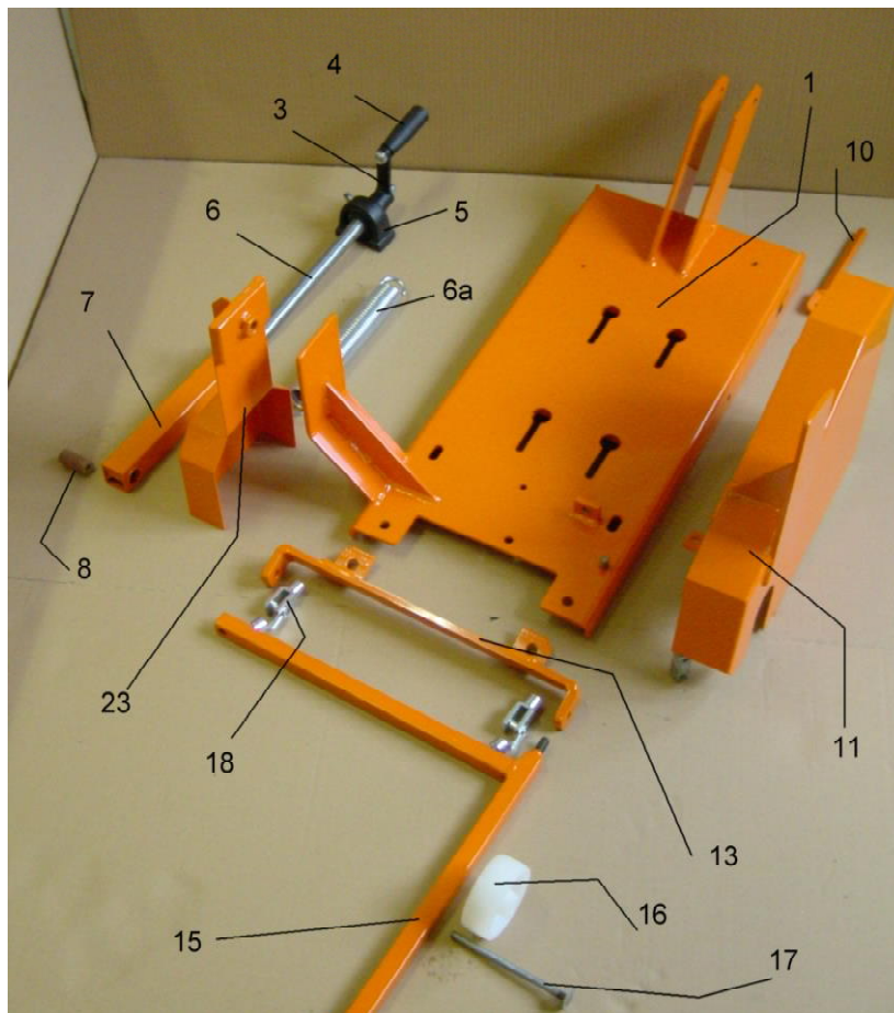
Wippenplatte mit Tiefenverstellung
