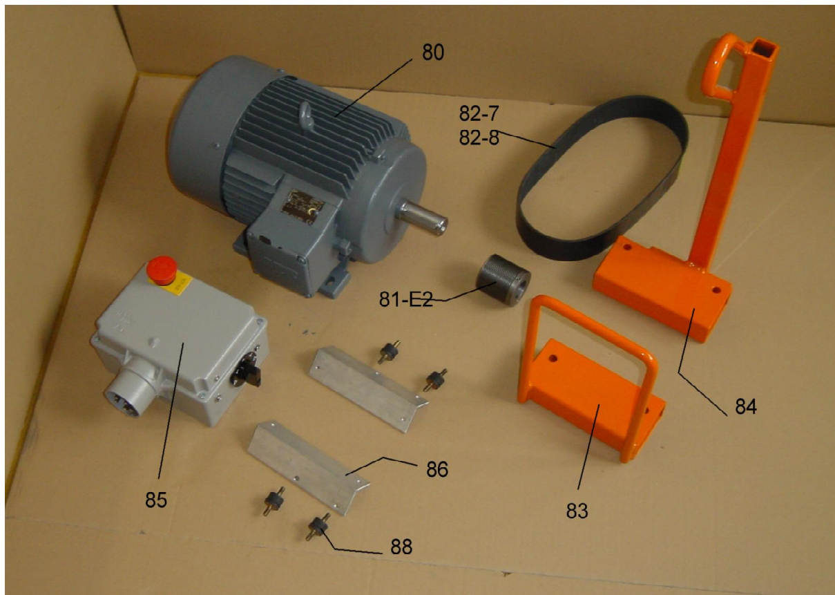
Elektromotor mit Schalter
