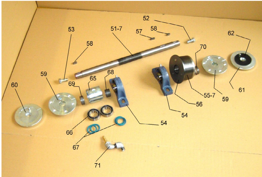
Schneidwelle mit Spülbüchse zu BS6E2-700
